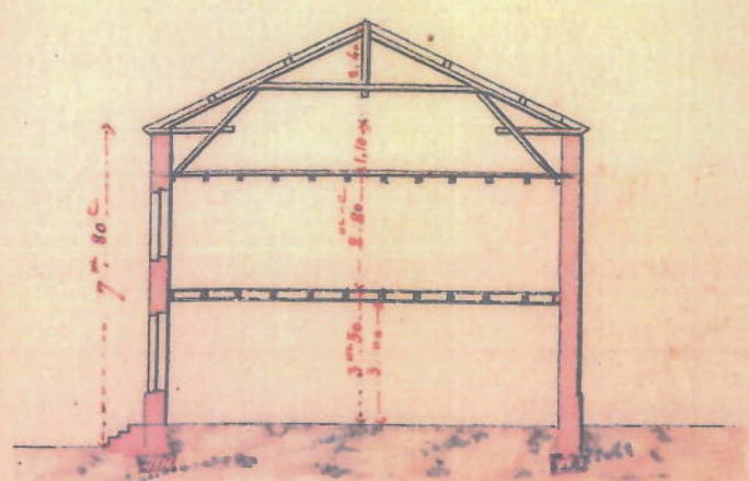
Coupe en Travers.
